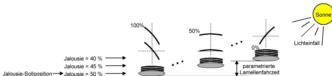
Bild 12: Beispiel für Lamellenpositionierung mit Auswirkung auf die Jalousieposition (Beispielhaft für Lamellentyp 1. Typ 2 sinngemäß gleich.)
