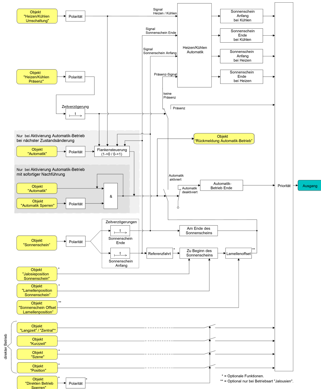
Bild 22: Funktionsschaltbild der Heizen/Kühlen-Automatik
