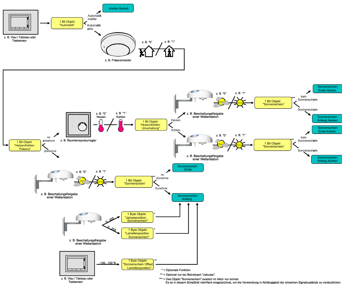
Bild 21: Prinzipschaltbild der Heizen/Kühlen-Automatik (zur Vereinfachung ohne Sperrfunktionen des Automatik-Betriebs oder des direkten Betriebs)
