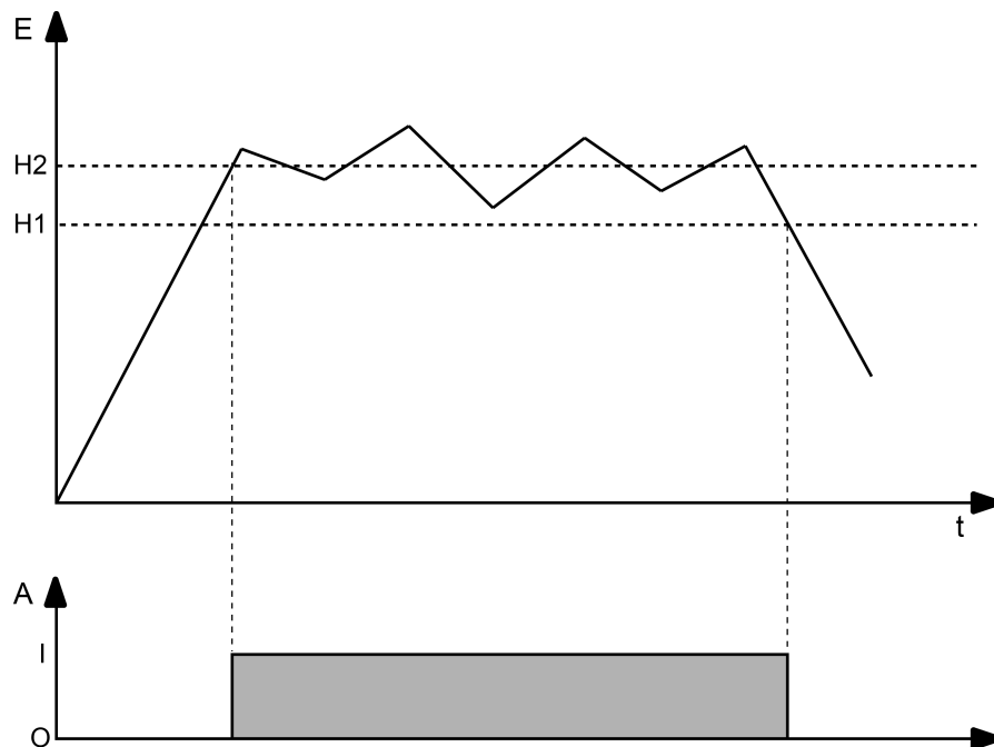
Bild 37: Beispiel einer Hystereseauswertung durch oberen und unteren Schwellwert
