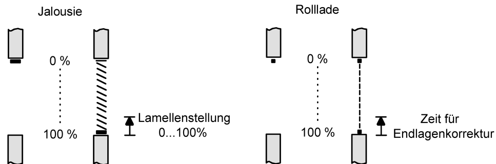
Bild 24: Endlagenkorrektur einer Jalousie oder Rolllade
