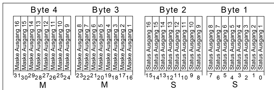
Bild 25: Struktur des Objekts "314" der Sammelrückmeldung für die Schaltausgänge 1...16
