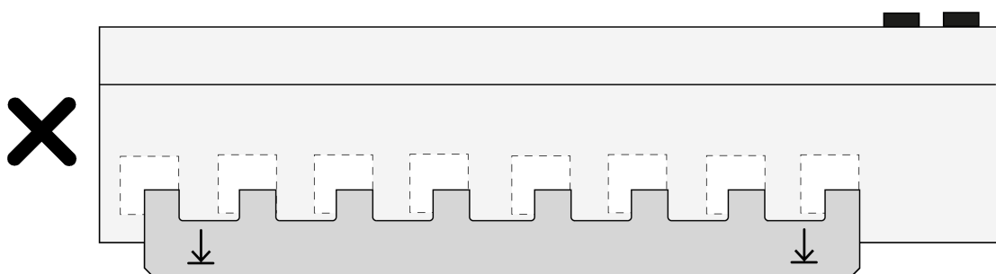
Bild 5: Phasenschiene montieren
