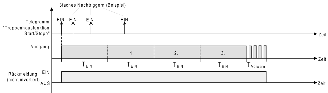
Bild 30: Zeitverlängerung der Treppenhausfunktion
