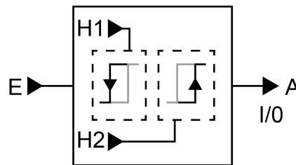
Bild 36: Grenzwertschalter
