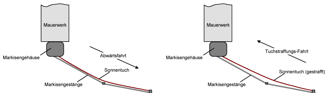
Bild 23: Tuchstraffung einer Markise
