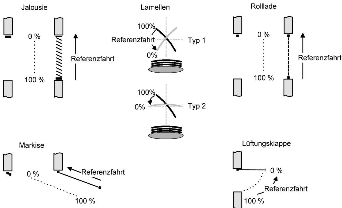
Bild 14: Referenzfahrt
