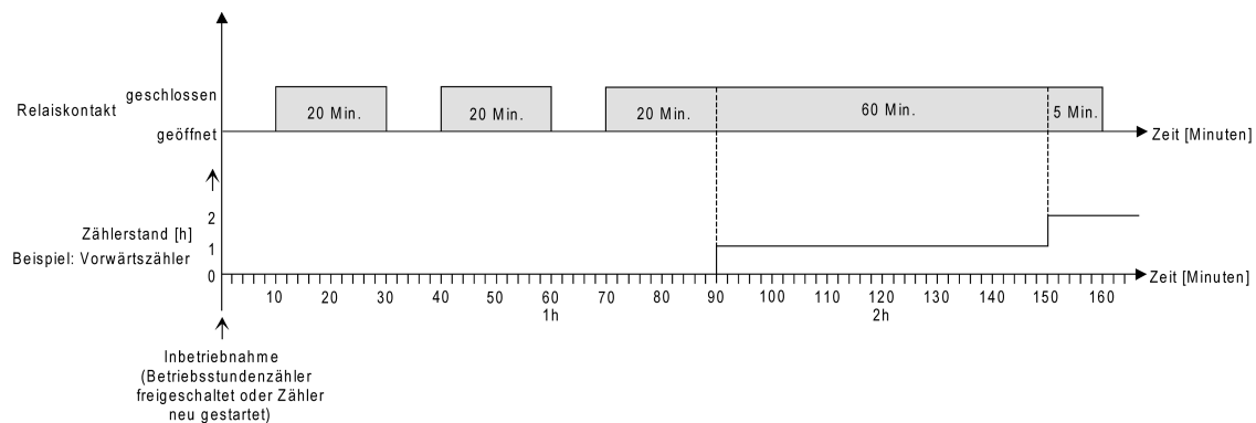
Bild 32: Funktionsweise des Betriebsstundenzählers (am Beispiel gezählter Stunden)
