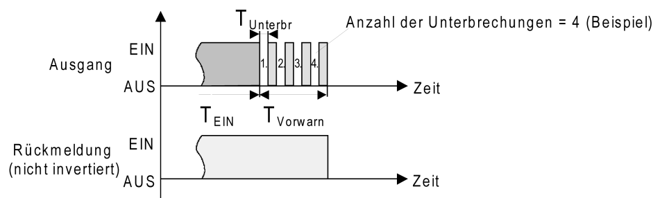
Bild 29: Die Vorwarnfunktion der Treppenhausfunktion (Beispiel)
