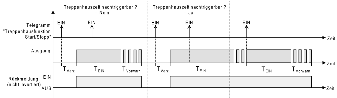
Bild 27: Einschaltverhalten der Treppenhausfunktion
