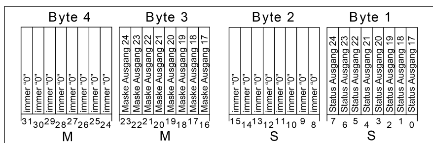
Bild 26: Struktur des Objekts "315" der Sammelrückmeldung für die Schaltausgänge 17...24
