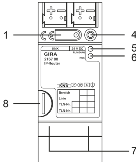
Abbildung 3: KNX IP-Router
