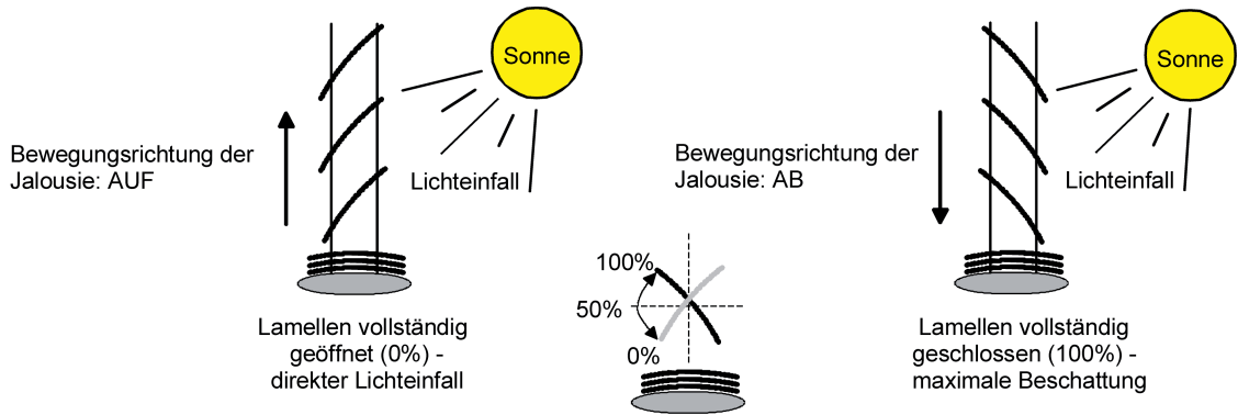
Bild 12: Typ 1 - Lamellenjalousien mit schräger Lamellenstellung in beide Fahrrichtungen
