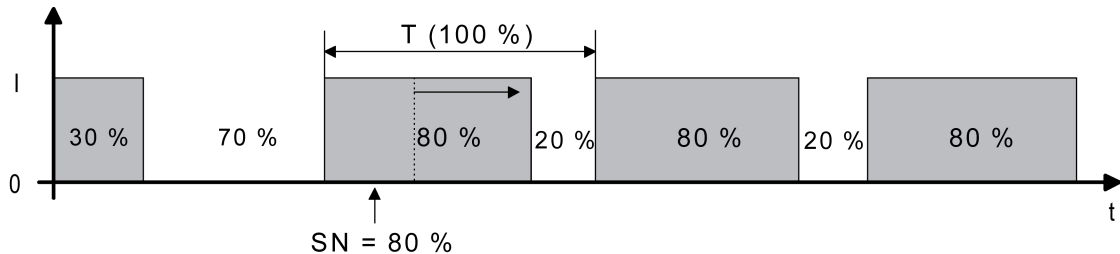
Bild 43: Stellgrößenänderung z. B. von 30 % auf 80 % während Öffnungsphase des Ventils
