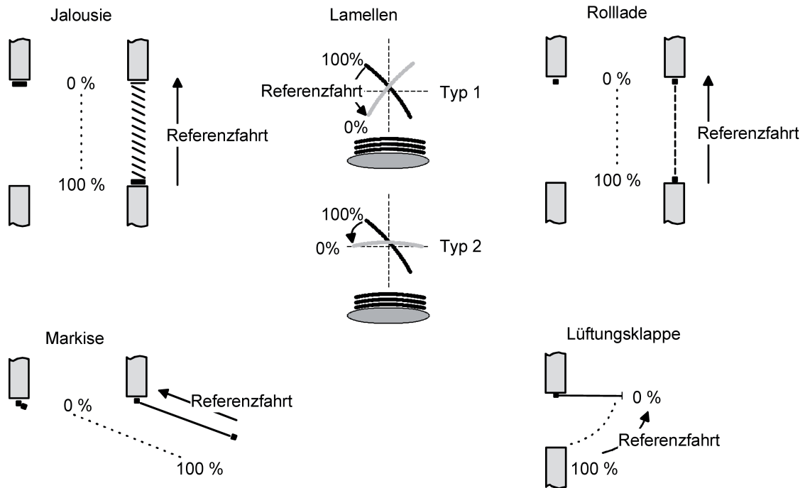
Bild 17: Referenzfahrt
