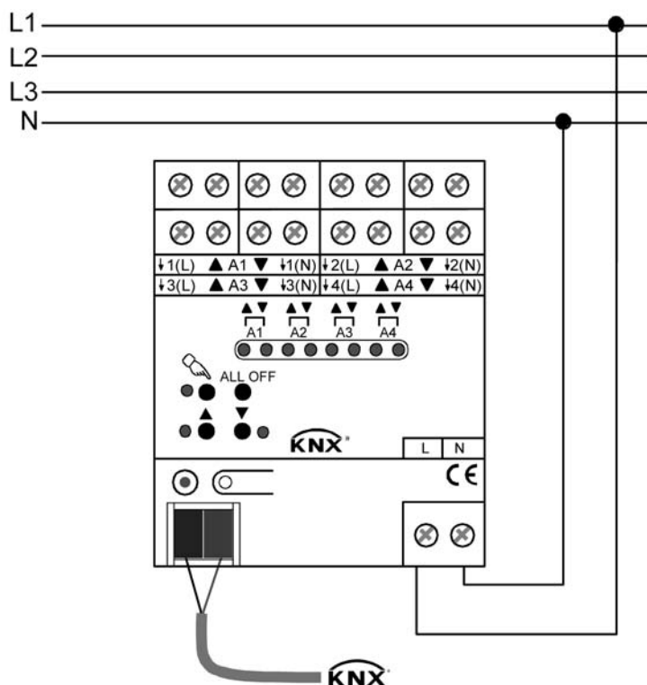
Bild 2: Elektrischer Anschluss der Netzspannungsversorgung und der Busleitung
