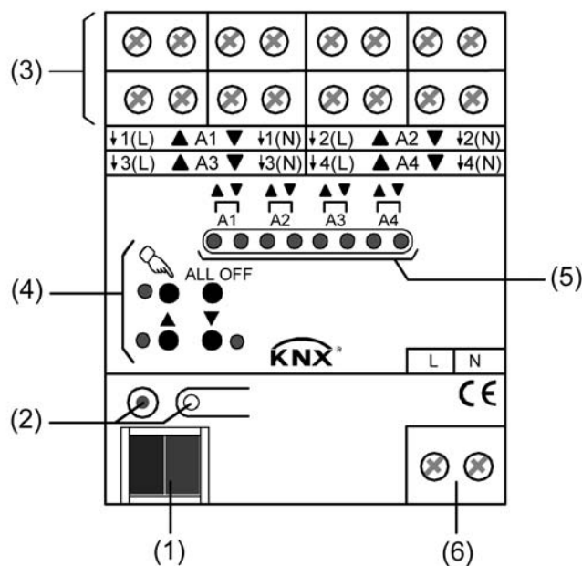
Bild 1: Geräteaufbau
