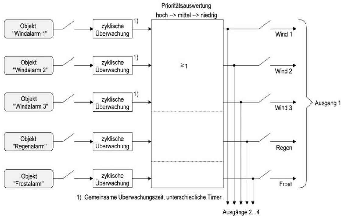
Bild 6: Funktionsschaltbild der Sicherheitsfunktionen
