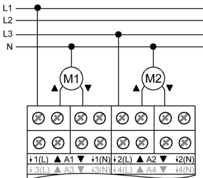
Bild 3: Elektrischer Anschluss für 230 V-Antriebsmotoren
