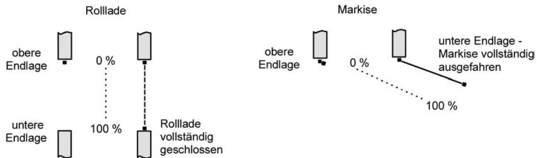
Bild 8: Positionsdefinition in Abhängigkeit der Antriebsart
