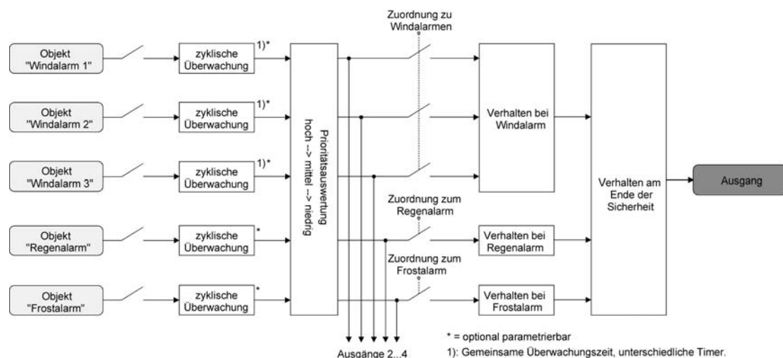
Bild 10: Funktionsschaltbild der kanalorientierten Sicherheitsfunktionen
