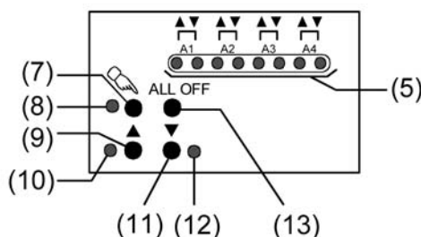
Bild 5: Bedien- und Anzeigeelemente der Handbedienung an der Gerätefront
