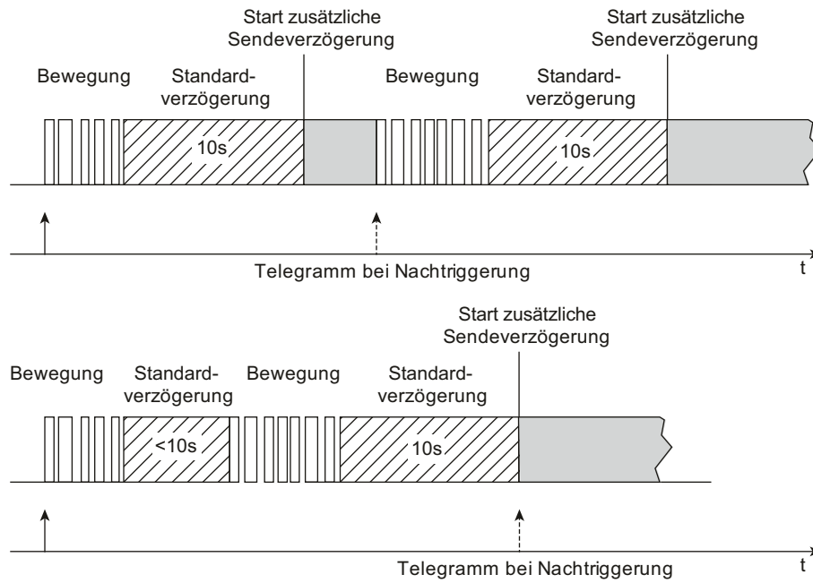
Bild 44: Telegrammauslösung bei Nachtriggerung
