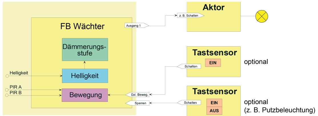
Bild 23: Applikationsbeispiel der Anwendung Wächter
