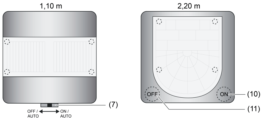
Bild 32: Anordnung der Bedienelemente zur Vor-Ort-Bedienung (Betriebsartenumschaltung)
