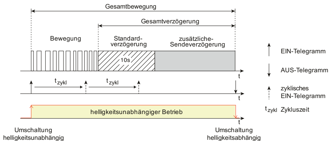
Bild 42: Gesamtbewegung mit Bewegungserfassung, Standardverzögerung und zusätzlicher Sendeverzögerung
