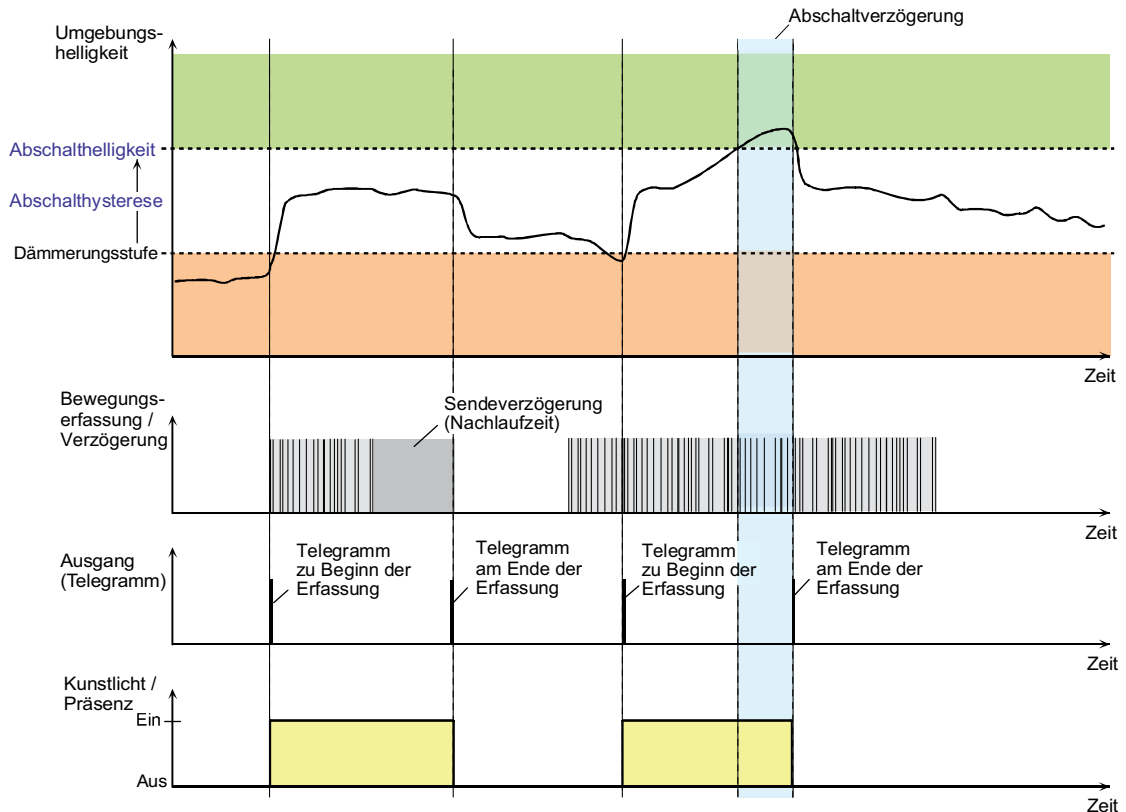
Bild 26: Helligkeits- und Bewegungsauswertung beim Wächter mit Abschalthelligkeit
