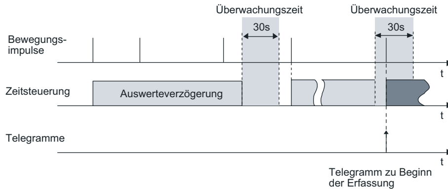
Bild 46: Auswertverzögerung mit nur kurzzeitiger Bewegung
