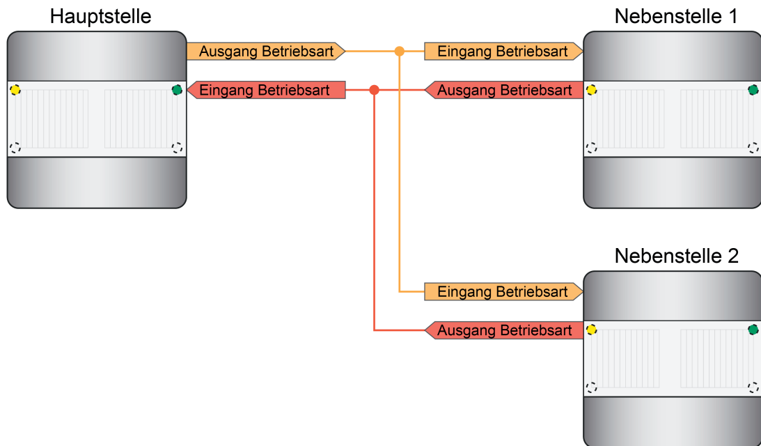
Bild 34: Beispiel zur Verknüpfung einer Hauptstelle mit zwei Nebenstellen zur Betriebsartenumschaltung und -anzeige
