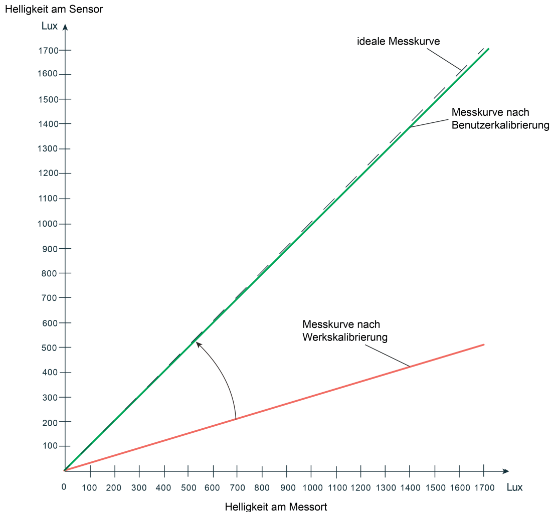
Bild 22: Messkennlinie nach Benutzerkalibrierung (Korrektur des Sensormesswerts auf die Umgebungshelligkeit = ideale Messkennlinie)
