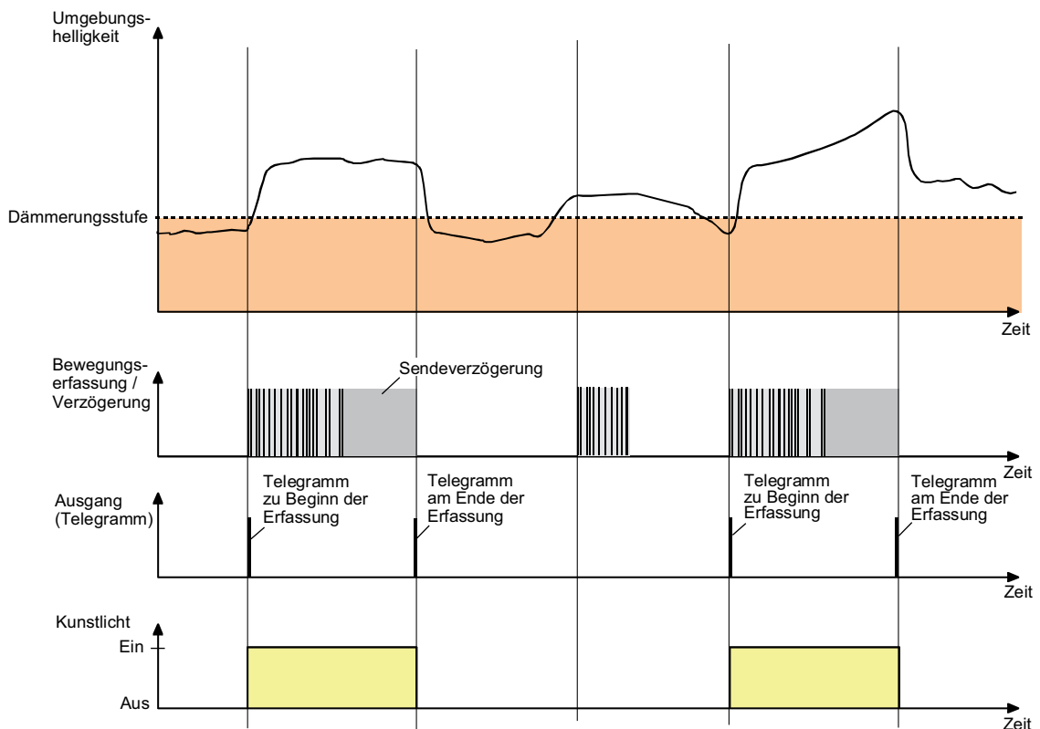
Bild 24: Helligkeits- und Bewegungsauswertung beim Wächter
