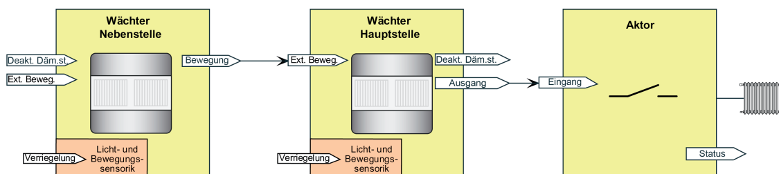
Bild 41: Applikationsbeispiel ohne Dämmerungsstufenauswertung in der Hauptstelle und in den Nebenstellen für Ausgangsfunktionen "Temperaturwertgeber" und "Betriebsmodus Raumtemperaturregler"
