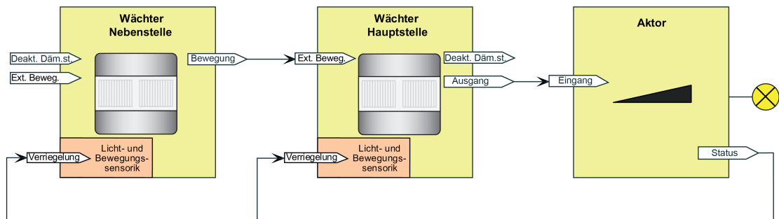
Bild 37: Applikationsbeispiel Haupt- und Nebenstelle mit Dämmerungsstufenauswertung in der Hauptstelle
