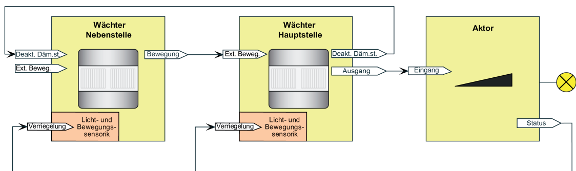
Bild 39: Applikationsbeispiel mit Dämmerungsstufenauswertung in der Hauptstelle und in den Nebenstellen Universal-Lösung für alle Datenformate
