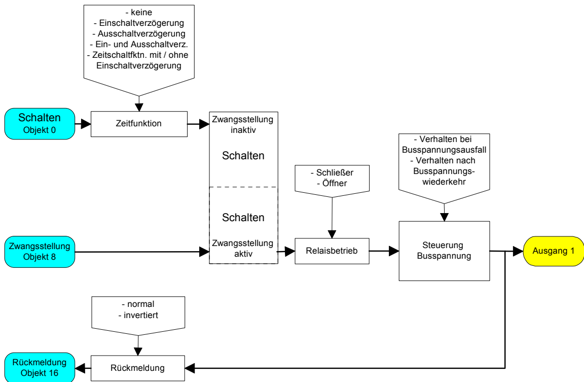
Funktionsschaltbild (für Schaltausgang mit der Zusatzfunktion "Zwangsstellungsobject")
