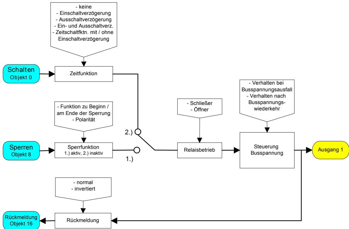
Funktionsschaltbild (für Schaltausgang mit der Zusatzfunktion "Sperrobject")
