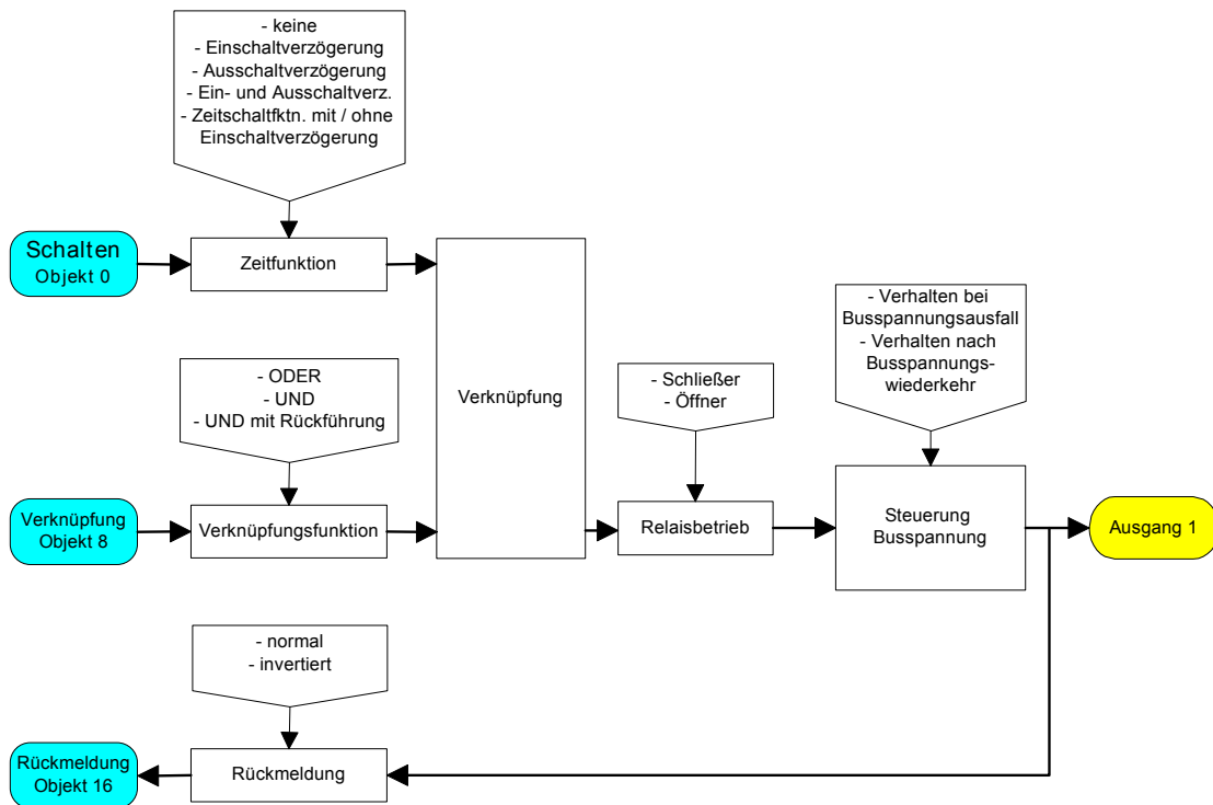
Funktionsschaltbild (für Schaltausgang mit der Zusatzfunktion "Verknüpfungsobjekt")
