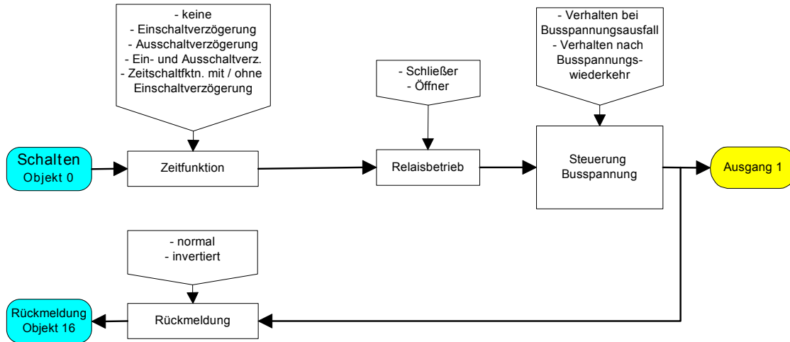
Funktionsschaltbild (für Schaltausgang ohne Zusatzfunktion)
