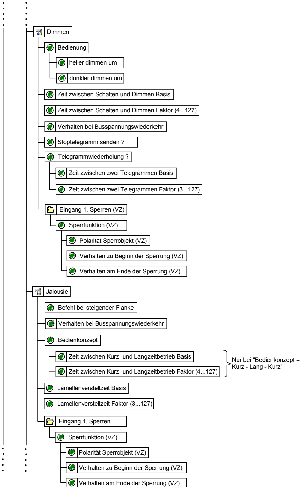
Parameterbild (Bild 4 von 6)
