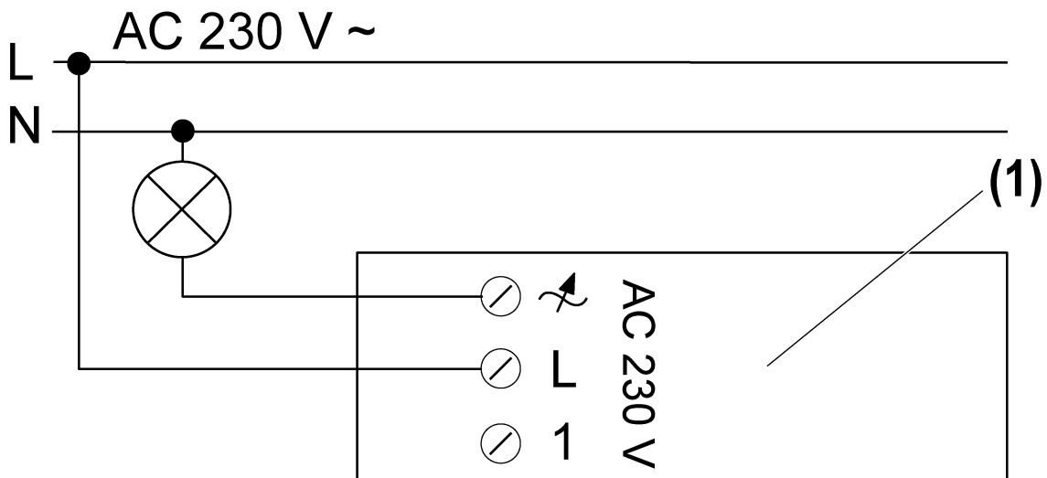
Imagen 3: Plano de conexión del regulador de luz
