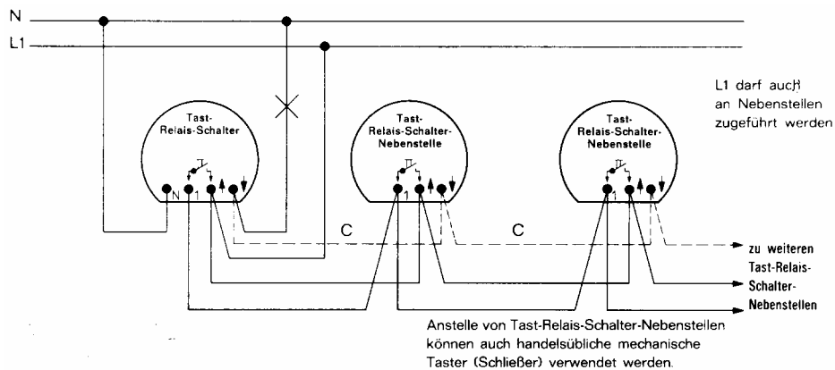
Tast-Relais-Schalter (Kreuzschaltung)
