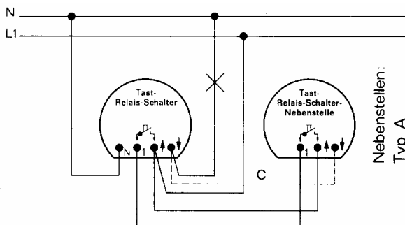
Tast-Relais-Schalter (Wechselschaltung)
