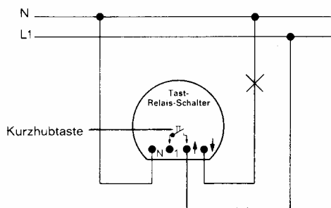
Tast-Relais-Schalter (Ausschaltung)
